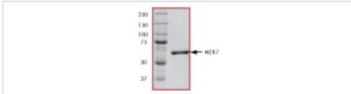
ab60703 on SDS-PAGE, MW ~63kDa.
